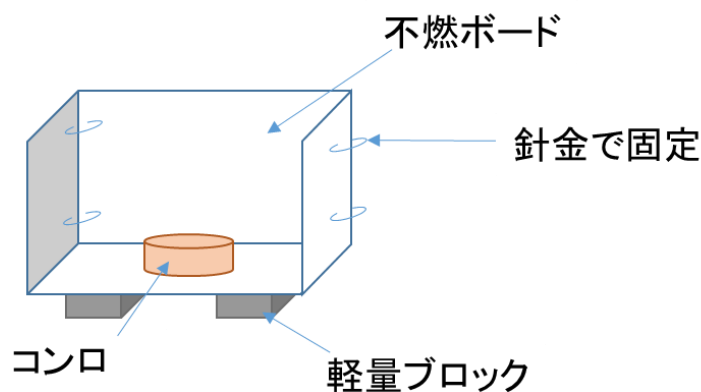
図 1 不燃ボードの組立図
