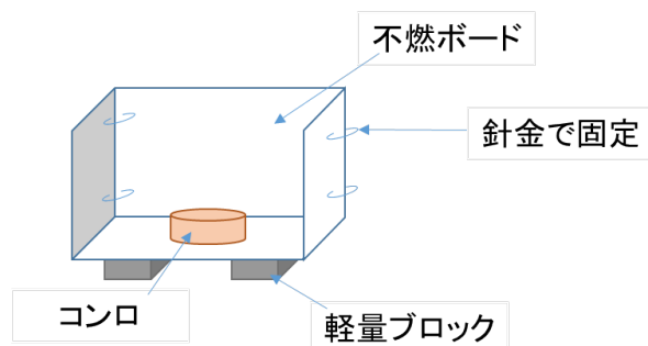
図 5. 不燃ボード組立図
