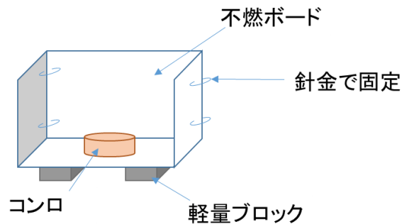
図 1 不燃ボード組立図
